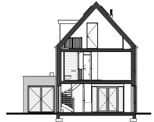
DOORSNEDE
