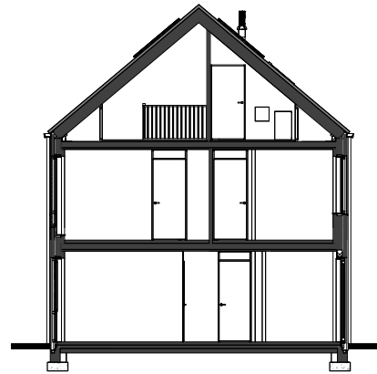
DOORSNEDE A
