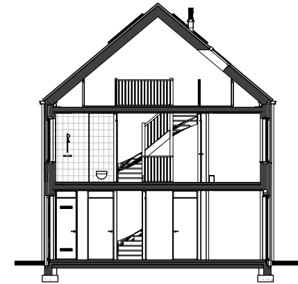
DOORSNEDE B
