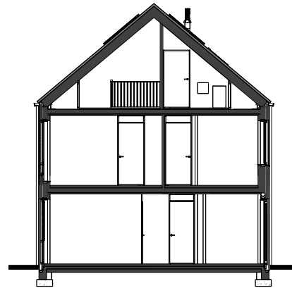
DOORSNEDE A
