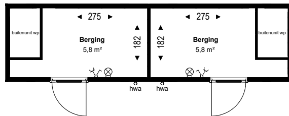
Begane Grond
